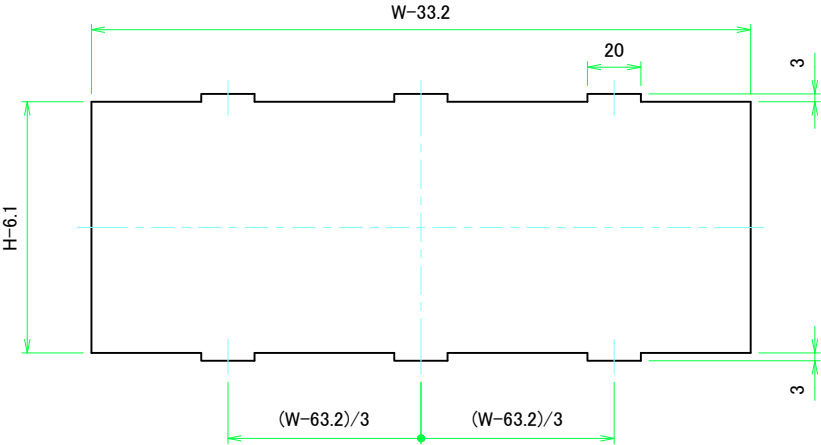
Wパネル1表面 / W Panel 1 Frontside
